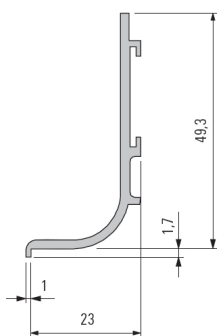
L-formos profilis (6 m) art.901014
